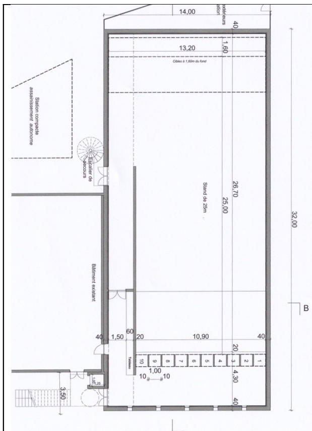
Plan au sol du 25m, RDC
