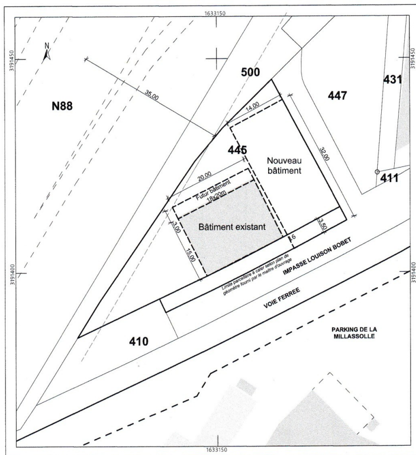
0. Plan de masse 1:500
