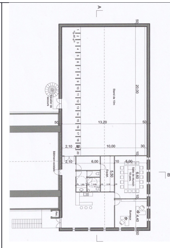
Plan au sol du 10m, 1er étage
